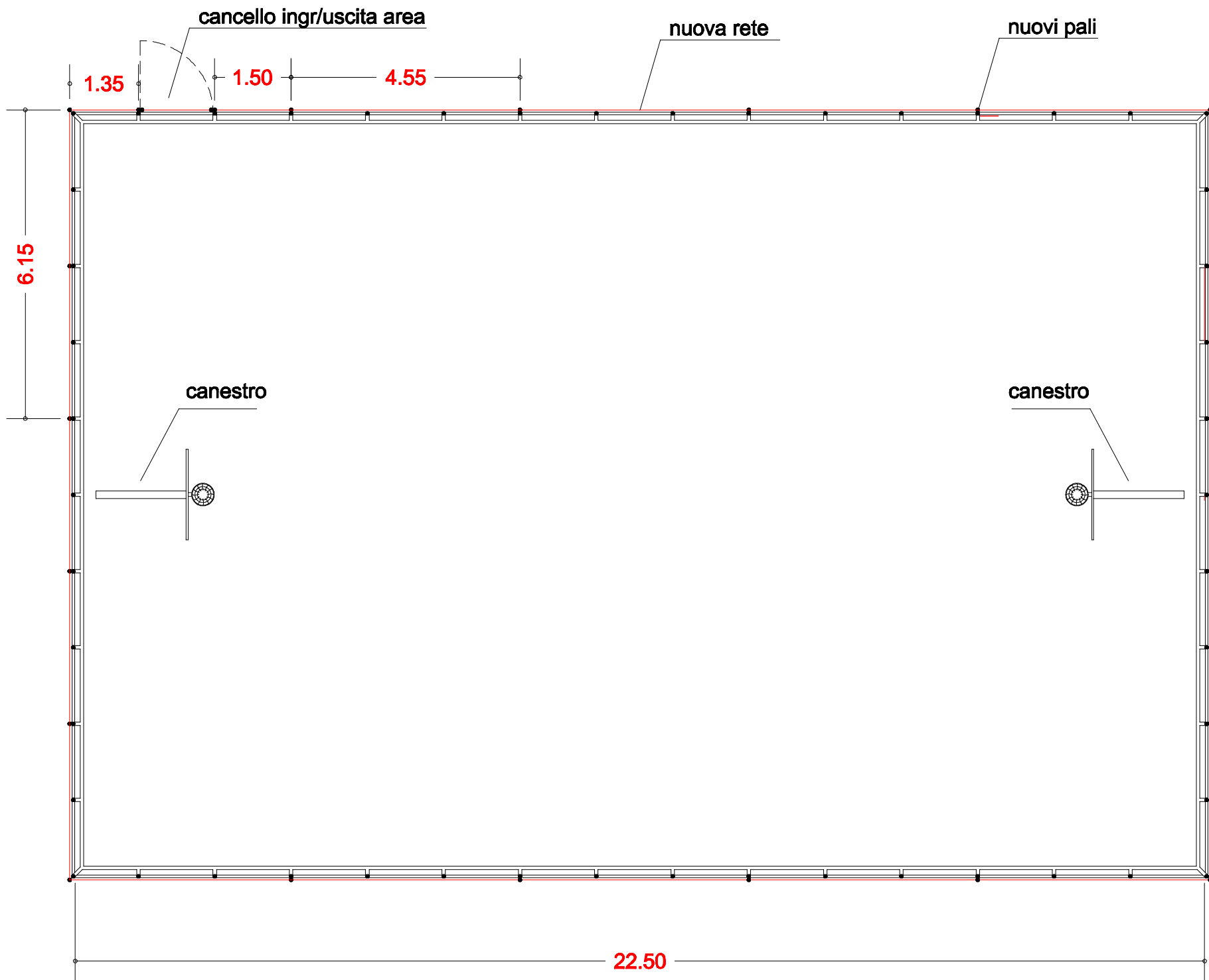
PIANTA STATO MODIFICATO 1/100
